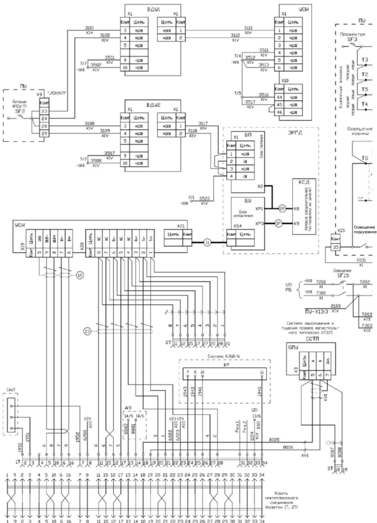
Рис. П5. Схема освещения тепловоза.
