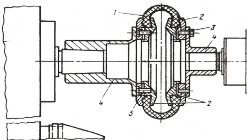
Рис.102. Муфта осевого вентилятора:
