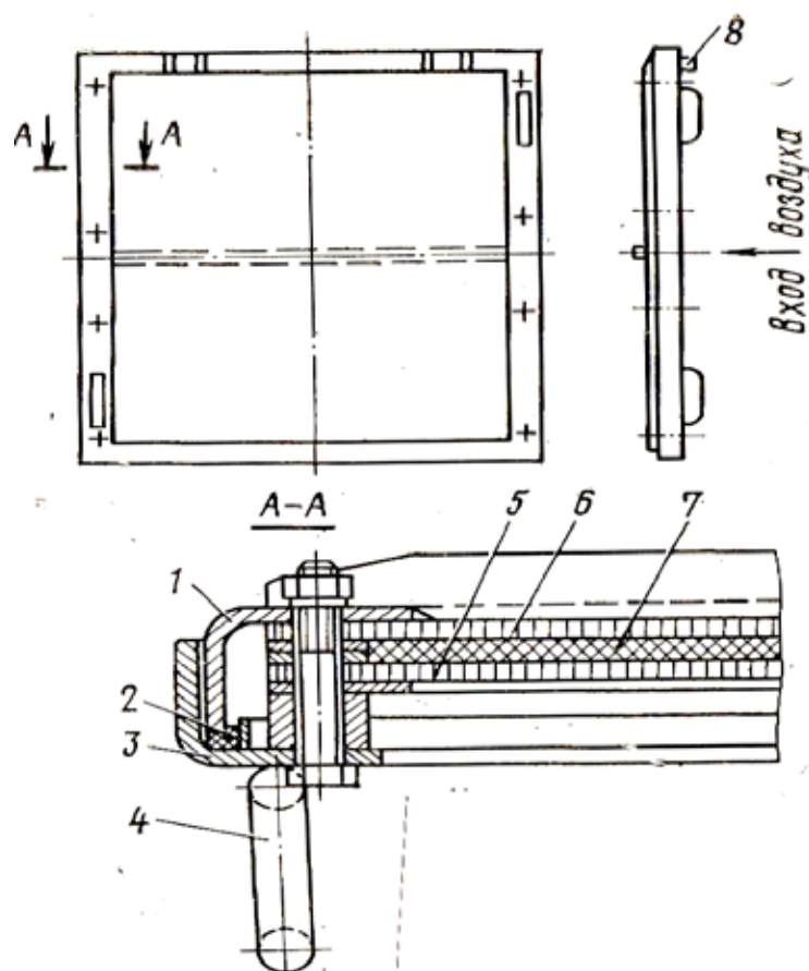
Рис.101(б). Кассета воздухоочистителя:
