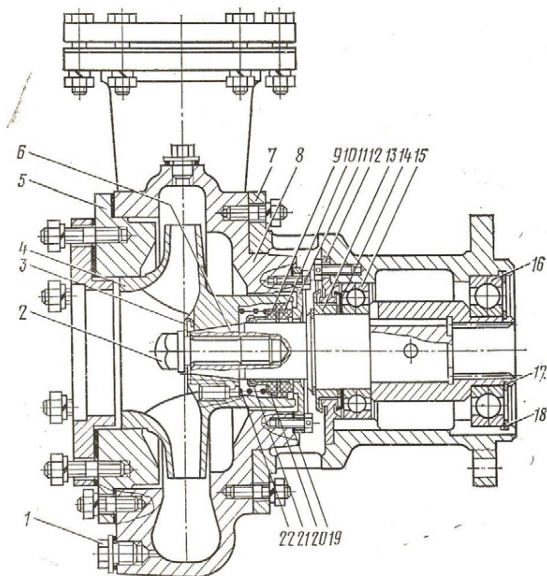
Рис.88. Водяной насос:
