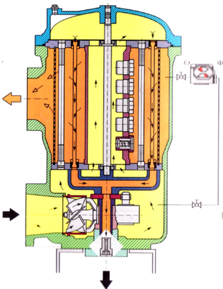
Рис.84б).Фаза обратной промывки
