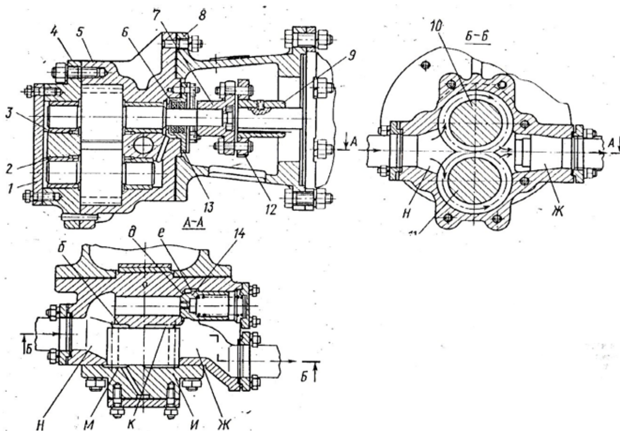
Рис.79. Насос маслопрокачивающий:
