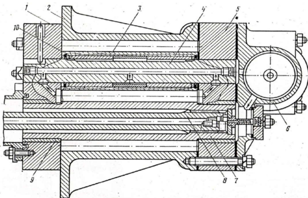
Рис.78. Главный масляный насос дизелей 16ЧН:
