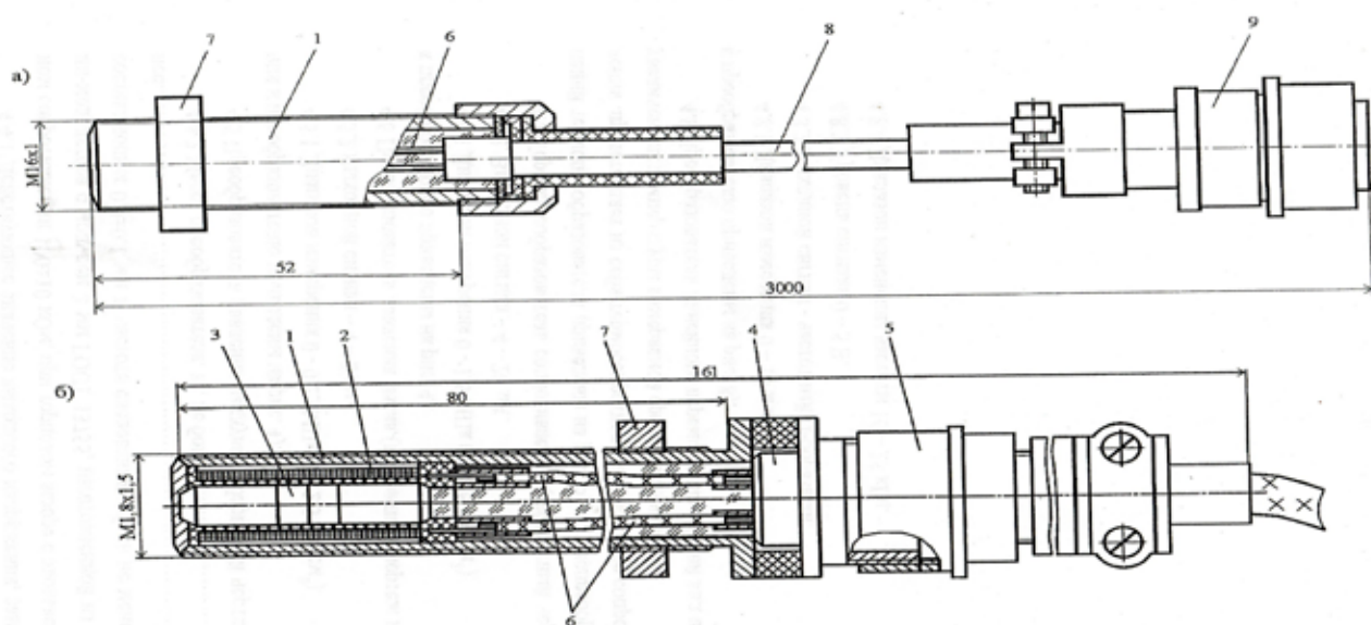
Рис.40. Преобразователи частоты вращения
