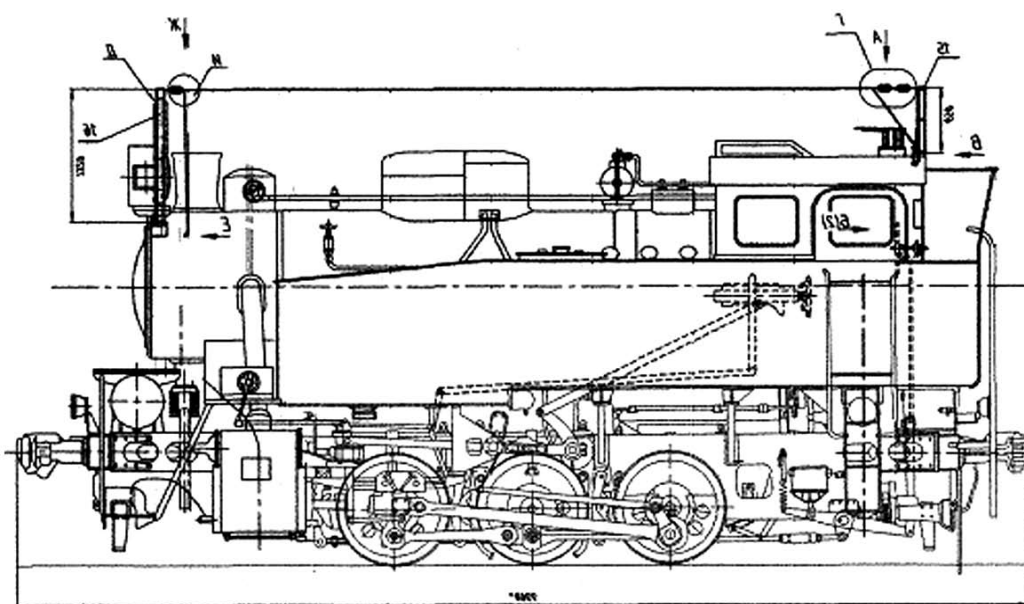
Рис. 295а. Размещение радиостанции РВС-1 на паровозе серии 9П
