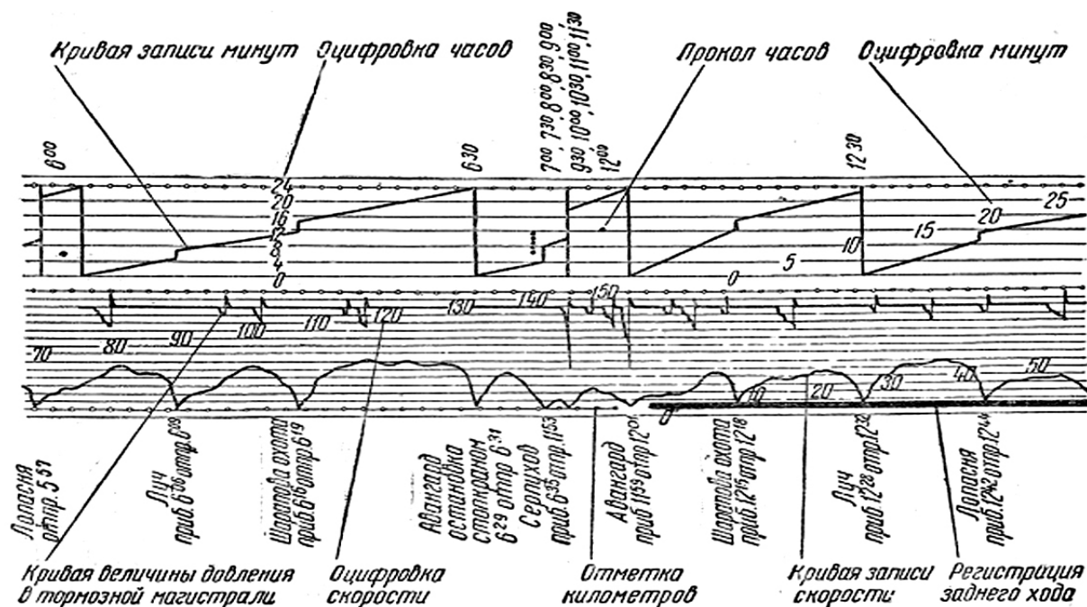
Рис. 291. Диаграмная лента
