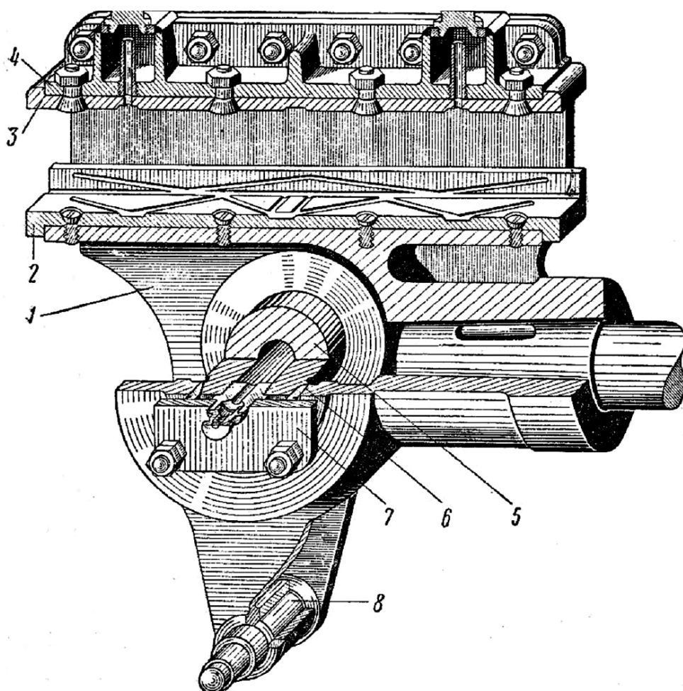
Рис. 136. Ползун паровоза серии СО: 1 – корпус; 2 – вкладыш бронзовый; 3 – рабочая поверхность вкладыша; 4 – крышка; 5, 8 – валик; 6 – разрезная втулка; 7 – планка нажимная
