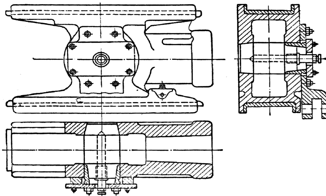
Рис. 137. Ползун паровоза серии Су
