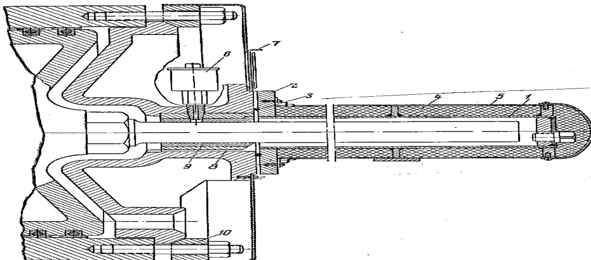
Рис. 124. Глухой сальник: 1 – чехол-футляр; 2 – фланец; 3 – кольцо обоймы, прокладное; 4 – асбест; 5 – обшивка; 6 – маслёнка; 7 – крышка; 8 – паз; 9 – втулка; 10 – кольцо
