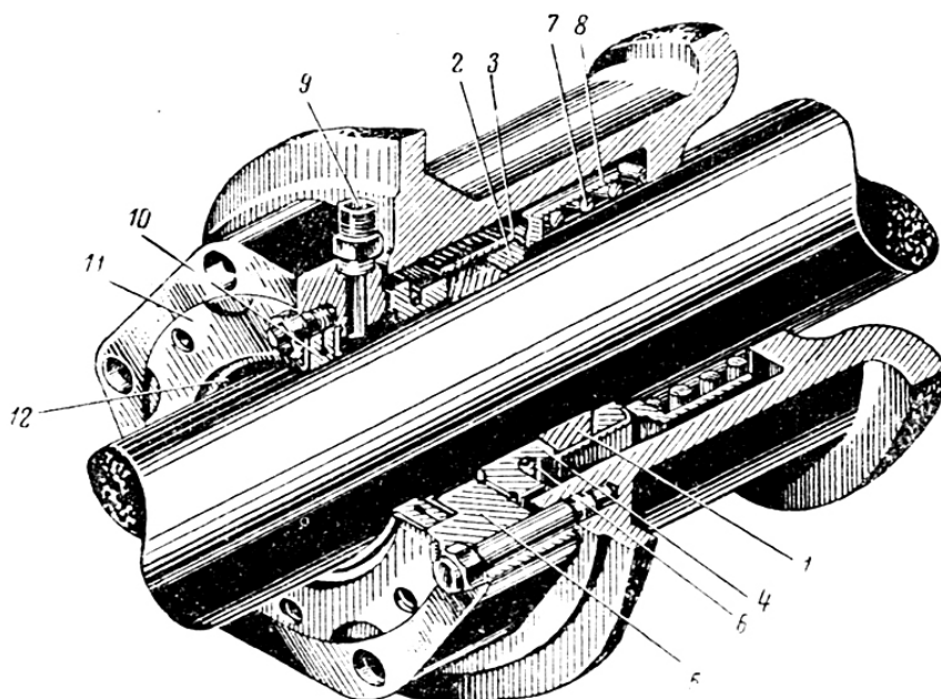
Рис. 122. Однокольчатый сальник: 1 – уплотнительное кольцо; 2 – кольцо нажимное; 3 – обойма; 4 – кольцо разрезное; 5, 6 – крышки сальника; 7 – пружина; 8 – стакан; 9 – штуцер; 10 – кольцо защитное; 11 – фланец; 12 – кольцо латунное разрезное
