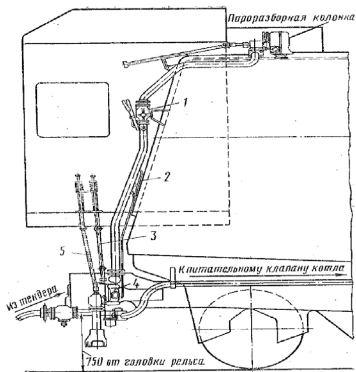
Рис. 80. Установка на паровозе ФД невосасывающего инжектора Н-400: 1 – паровой пусковой клапан; 2 – сигнальная трубка; 3 – привод к водяному клапану; 4 – инжектор; 5 – привод к вестовому клапану
