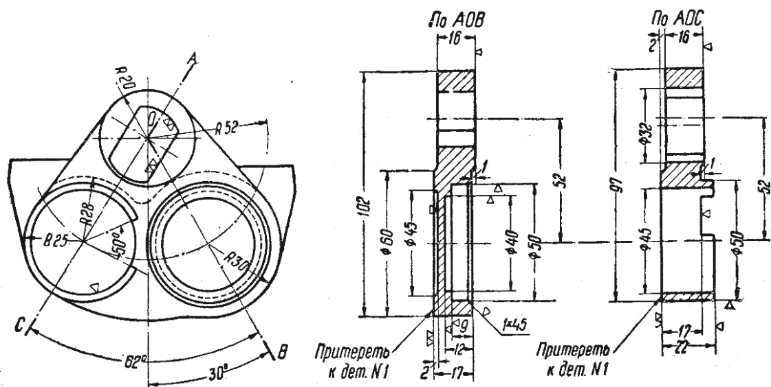
Рис. 72а. Рычаг заслонки спускного крана топки
