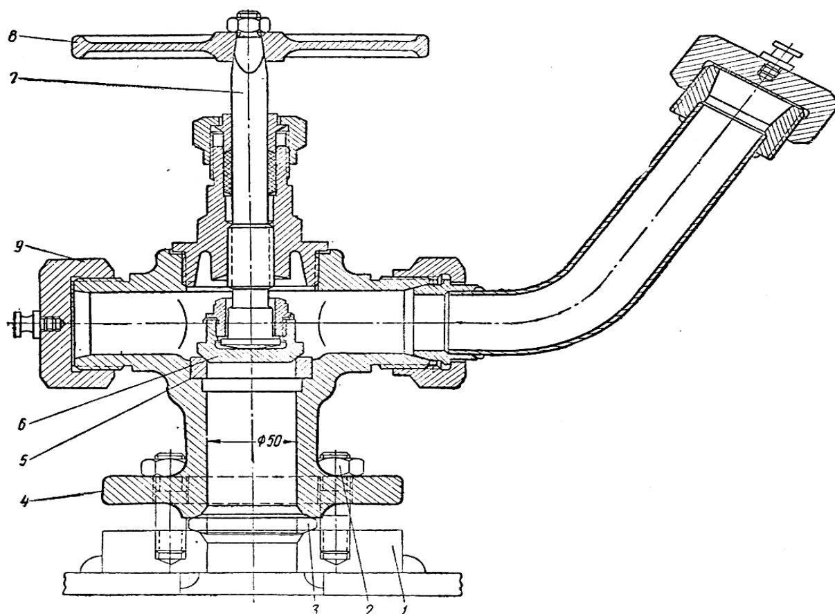
Рис. 73. Унифицированный вентиль тёплой промывки: 1 – фланец; 2 – шпилька; 3 – кольцо; 4 – вентиль; 5 – втулка-седло; 6 – клапан; 7 – стержень; 8 – ручка; 9 – гайка
