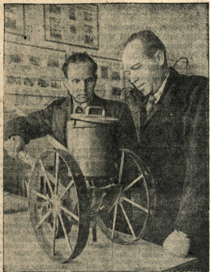
Всесоюзный научно-исследовательский институт лесного хозяйства сконструировал ручную селку для посева семян лиственных и хвойных пород в лесных питомниках. Производительность лесной селки—2 тысячи погонных метров в час. Обслуживается она одним рабочим. Завод «Рязельмаш» уже освоил массовый выпуск этих селок. На снимке: научные сотрудники института кандидат технических наук Ф. М. Курушин (справа) и инженер С. Г. Русаков осматривают промышленный образец лесной селки, полученный с завода «Рязельмаш». Фото В. Шаровского.
