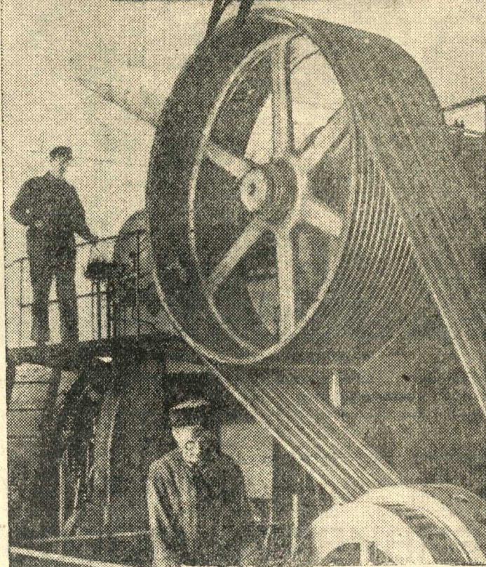
На ремонтно-механическом заводе построена электростанция. Она полностью обеспечит нужды завода в электроэнергии. На снимке: машинисты И. Истоин и В. Мурашов у локомобильной установки электростанции. Фото А. Говорова.
