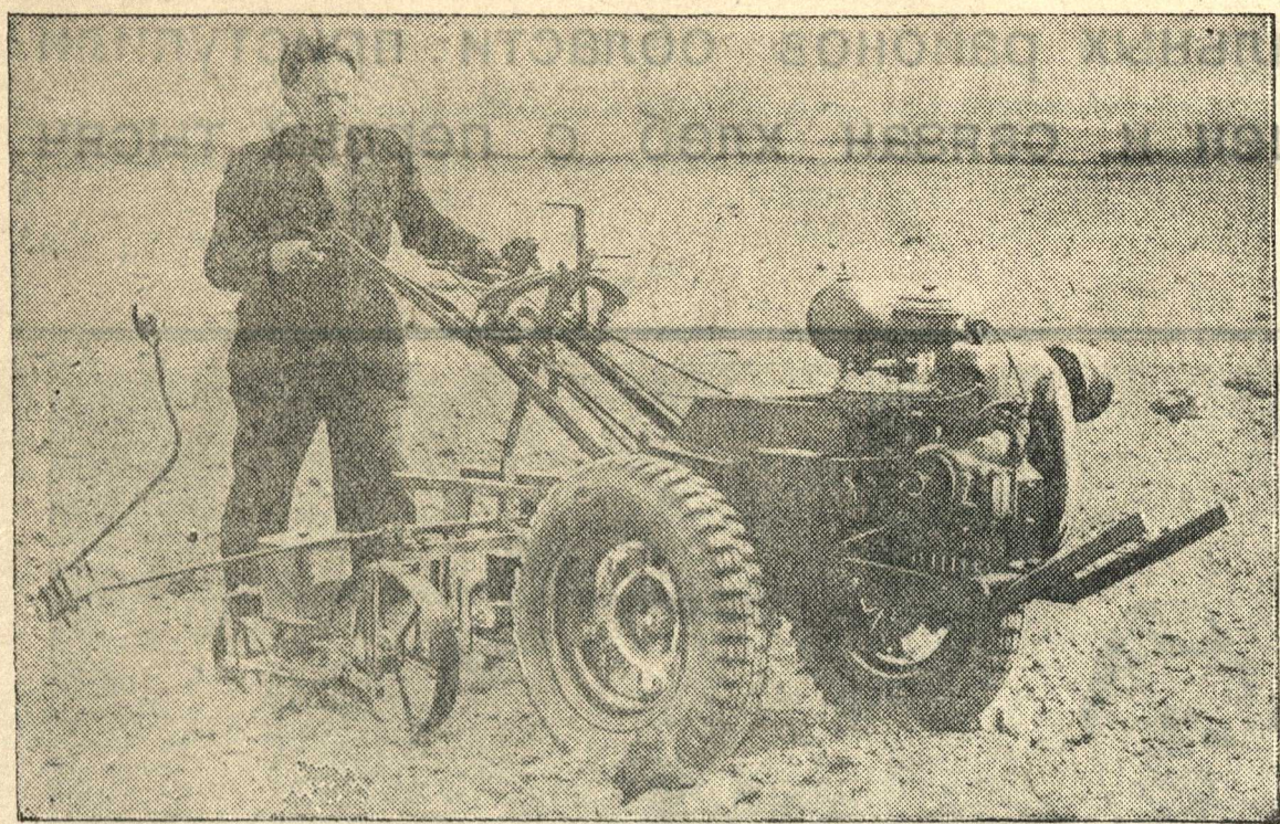
Инженеры Всесоюзного научно-исследовательского института сельскохозяйственного машиностроения (ВИСХОМ) М. Кузнецов, И. Курников, Н. Загребский и П. Котов сконструировали универсальный садово-огородный трактор. Основное назначение трактора — механизация работ при возделывании овощных, ягодных и технических культур. Кроме того, он применим для обработки садов, виноградных, чайных, табачных плантаций, а также для вспашки небольших земельных участков. Одновременно для трактора сконструирован набор навесных сельскохозяйственных машин и орудий: плуг, дисковая борона, два культиватора, полольник-рыхлитель и транспортная тележка на пневматическом ходу грузоподъемностью до 500 килограммов. На снимке: садово-огородный трактор. Управляет трактором инженер И. Курников.
