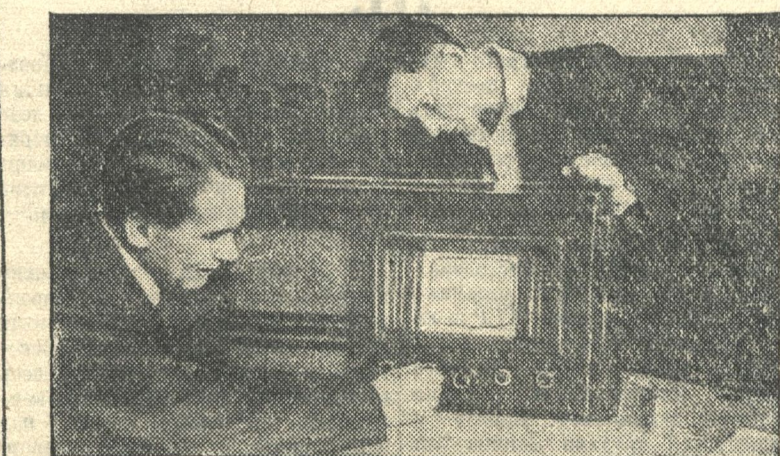
Ленинградский завод имени Козицкого осваивает производство индивидуальных телевизоров «Ленинград Т-1». Приемник компактен, прост в управлении. Изображение проектируется на экран размером 105 на 135 миллиметров. На снимке: проверка образца телевизора «Ленинград Т-1».
