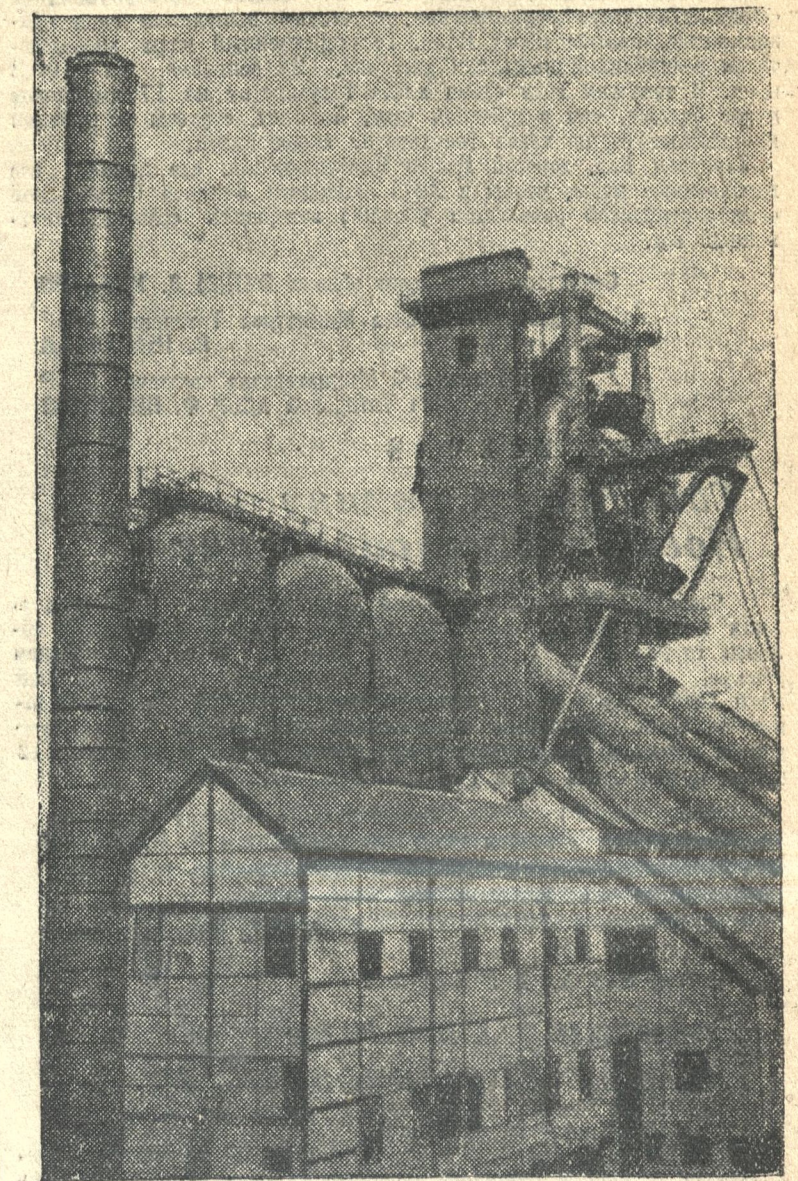
Доменная печь № 3 «Запорожстали»
