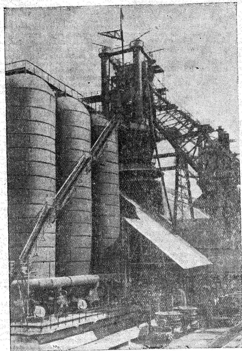
Воршиловск. На днях на металлургическом заводе имени Ворошилова вступила в строй крупная доменная печь. На снимке: общий вид восстановленной доменной печи № 1.
