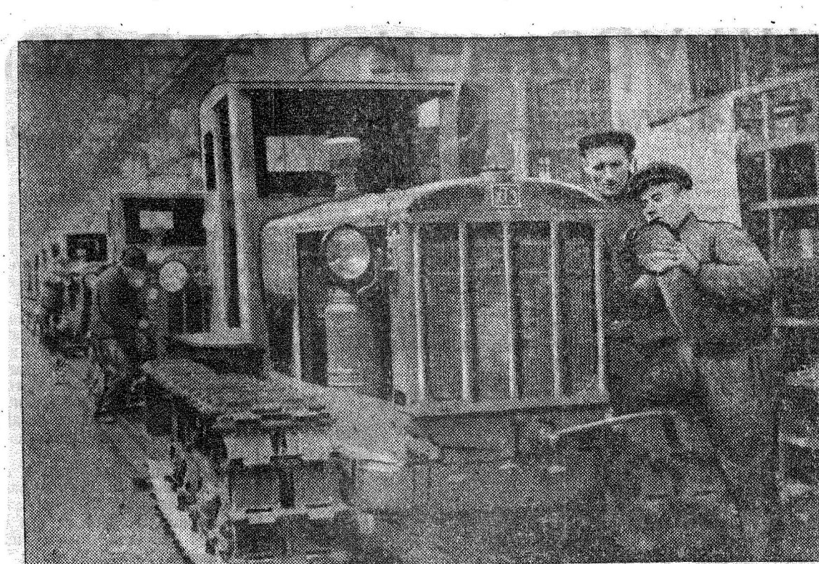
На Харьковском ордена Ленина тракторном заводе имени Орджоникидзе заканчивается восстановление вехущих цехов. Завод уже выпускает гусеничные тракторы «ХТЗ». На снимке: сборка тракторов на конвейере. На переднем плане — двухсоткишечный сменный мастер В. П. Замогильный и слесарь А. Т. Демченко. Фото Л. Леонидова.
