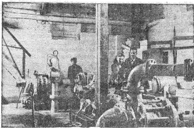
Главная насосная станция Курского водопровода. Общий вид машинного зала. Фото В. Строева.
