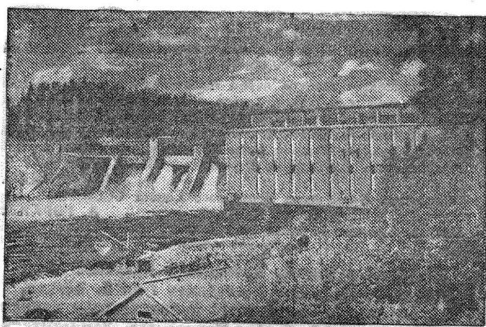
Гидроэлектростанция Раухина на реке Вуокса (Карельский перешеек). Фото Б. Васитинского.
