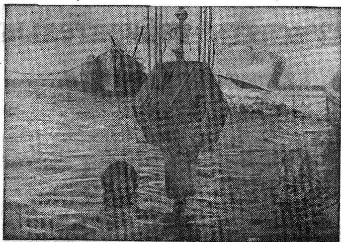
На восстановлении рейдового мола Одесского порта водолазы уложили под водой 6.000 кубометров бетона. На снимке: водолазы заделывают последний пролом.
