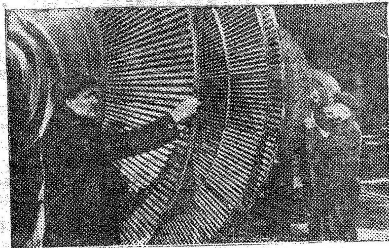
Осмотр ротора паротурбины на Ленинградском заводе, где директором тов. Кожаринов. Фото В. Капустина.
