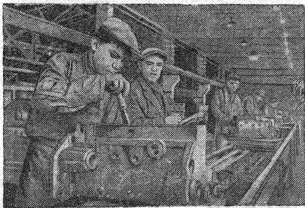
Поточная сборка токарных станков на Московском ордена Ленина станкостроительном заводе «Красный пролетарий». На переднем плане — слесарь сборщик А. И. Зотов, выполняющий сменное задание на 300 процентов.
