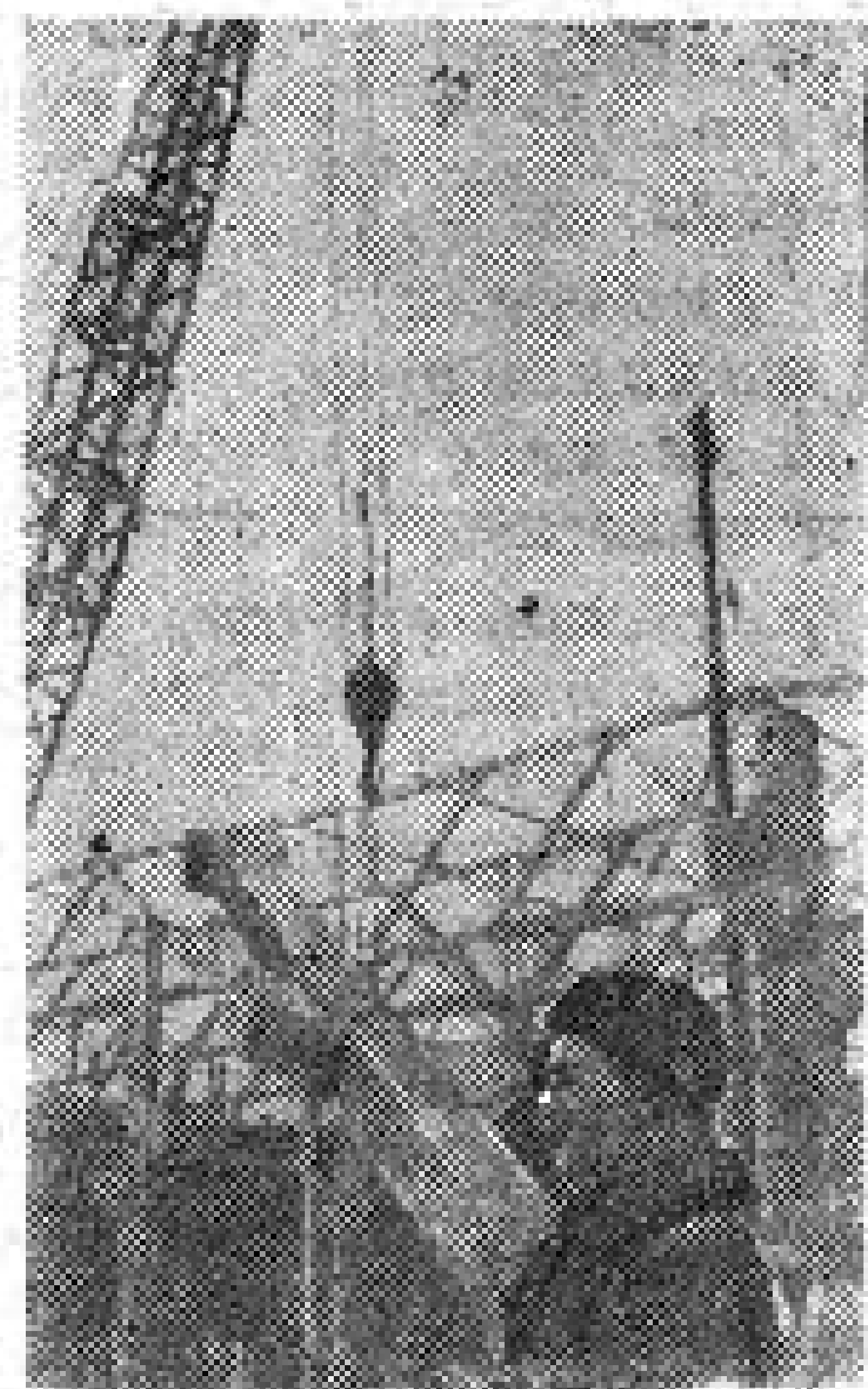
Скоростное строительство Н-ского завода. Монтаж основных конструкций механосборочного цеха. На переднем плане — знаменитый бригадир-монтажник И. В. Веседин, награжденный орденом «Знак почта». Фото С. Малебницкого.
