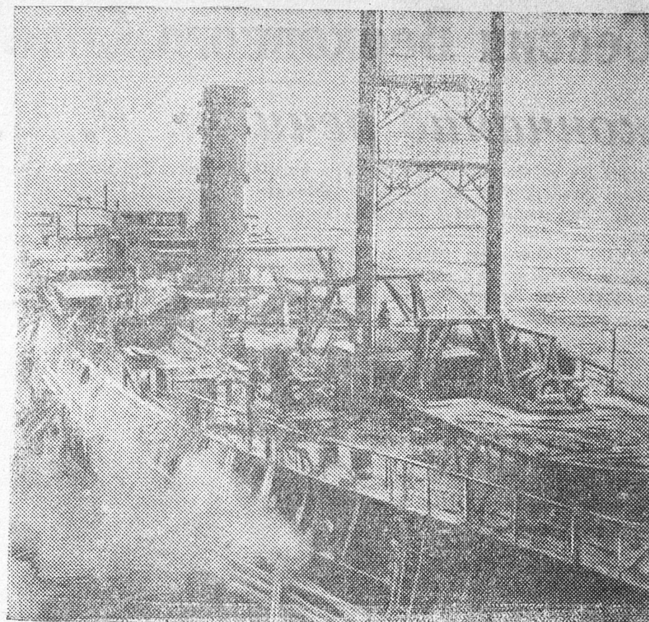
На ленинградском заводе имени Серго Орджоникидзе строится мощный ледокол «И. Сталин». Надвиг на ледоколе установлены греб-мачта и кормовая труба. На снимке: строительство ледокола «И. Сталин».
