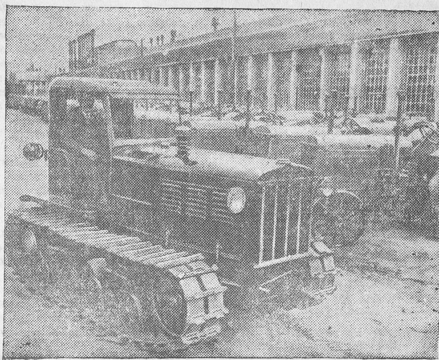
На Сталинградском тракторном заводе изготовлен гусеничный трактор «СТЗ-НАТИ» для международной Парижской выставки. На снимке: трактор «СТЗ-НАТИ» для Парижской выставки.
