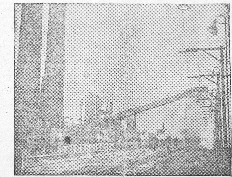
Введенная в строй в январе первая батарея неокисных печей нового комсомольского завода в Крыжме. Работает бесперебойно. На снимке: рабочая площадка второй батареи неокисных печей Крыжмского завода.
