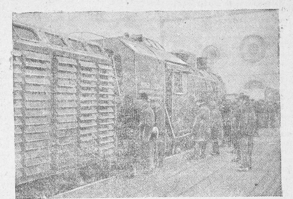
В Москву прибыл со станции Голутвино первый паровоз «Серго Орджоникидзе» с тендер-конденсатором, выпущенный Коломенским заводом. Этот новый тип паровоза, как заявил тов. Л. М. Каганович на декабрьском пленуме ЦК ВКП(б), совершит революцию в паровозном хозяйстве. Новый паровоз излучает отработанный пар и поэтому расходует воды в 20—25 раз меньше, чем обычный паровоз. Он может проходить 1000 км. без набора воды. На снимке: новый паровоз «О» у перрона московского вокзала Моск. ж. д. На переднем плане тендер-конденсатор.
