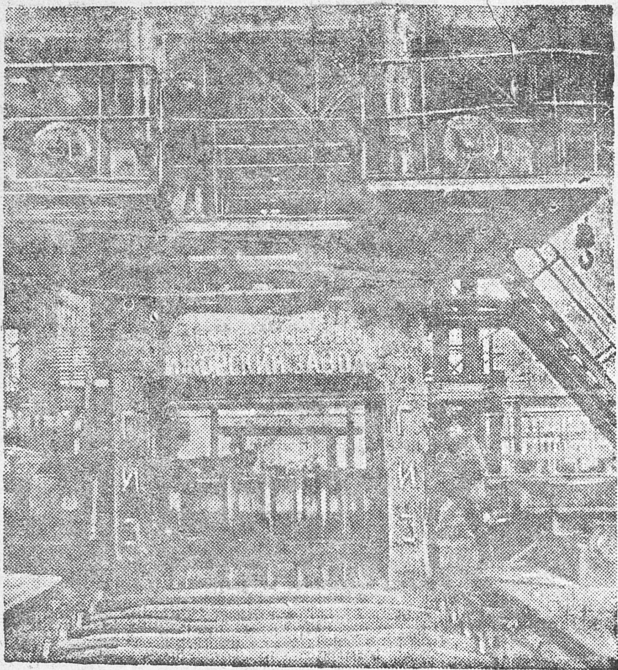
На Златоустовском металлургическом заводе закончен монтаж советского блюминга, построенного Ижорским заводом. К 1 января 1935 г. завод должен получить для своего проката первые блюмы. Мощность блюминга рассчитана на 720 тысяч тонн проката (блюмов) в год.
